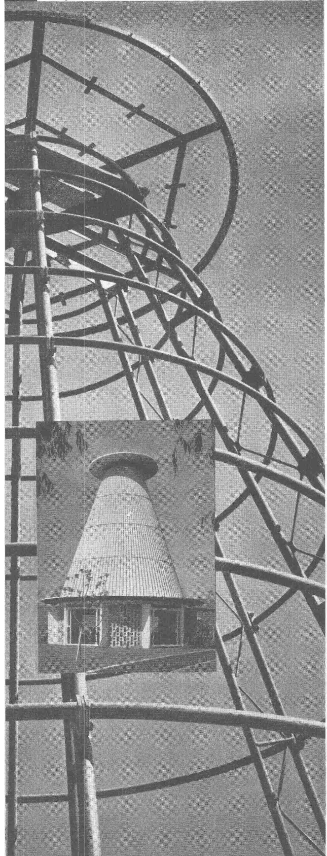
Teepavillon des Strandbades Tiefenbrunnen, Stahlskelett und fertiges Bauwerk
