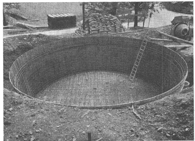
Schwerölbehälter 250 000 Liter
