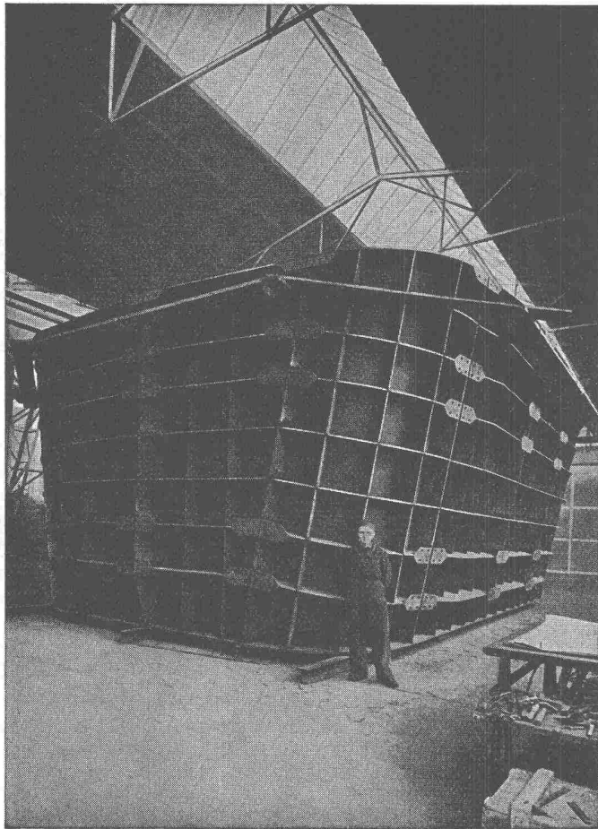
CUVE EXTÉRIEURE DE FOUR ÉLECTRIQUE POIDS 100 TONNES
