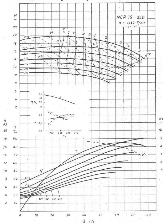
Kennlinien einer Spiralgehäusepumpe mit verschiedenen Laufraddurchmessern
