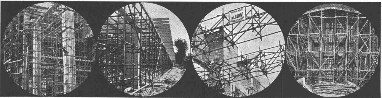
Schweres Stützgerüst
