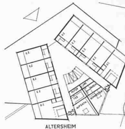
Altersheim, erstes Ober- geschoss, links Erdge- schoss, 1:900
