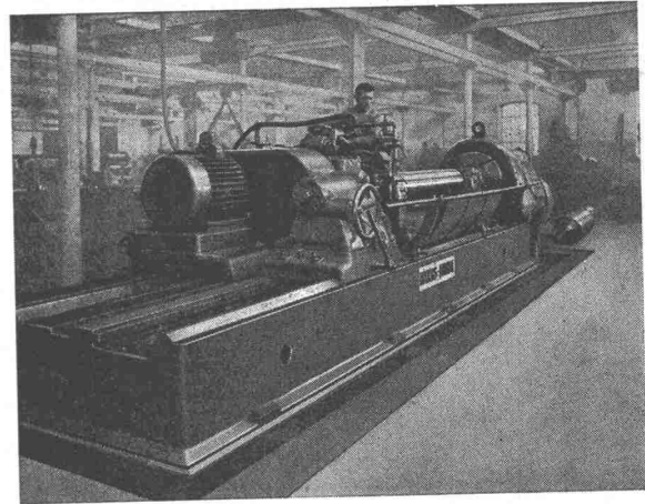
Isolierte Walzenschleifmaschine
