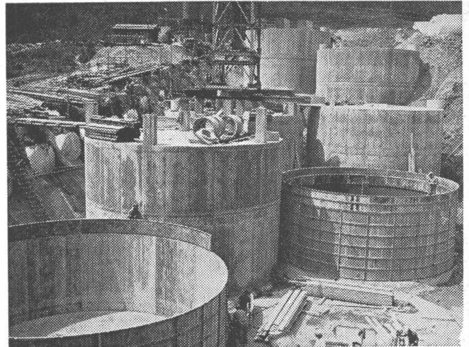
Migrol - 16 Tanks à je 500 000 Liter
