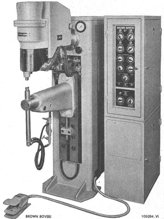
Universelle druckluftbetätigte und röhrengesteuerte Punkt-schweismaschine. Sie eignet sich gleichermaßen für das Einzelpunktschweissen hoher Qualität und auch zum Steppen und für kleinere Buckelschweissarbeiten. Die zugeordnete elektronische Steuerung erlaubt nicht nur die Funktionen Vorpresen, Schweissen, Nachpressen und Repetieren, sondern auch das Mehrimpulsschweissen. Zudem kann mit Schwellstrom, auch Modulation oder «slope control» genannt, geschweisst werden und der Schweißstrom durch Zündpunktverschiebung an den Ignitrons geregelt werden.
