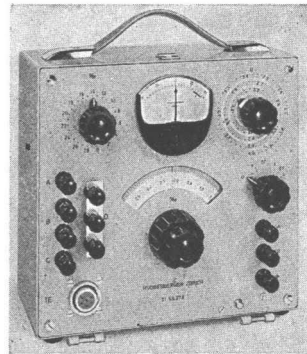
Volltransistor. Präzisions-Messbrücke
