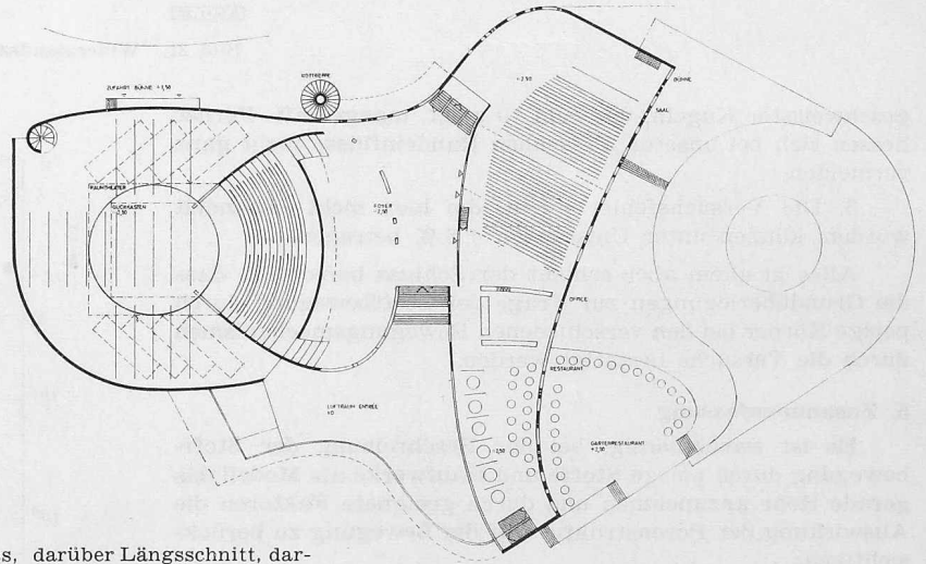
Hauptgeschoss, darüber Längsschnitt, darunter Erdgeschoss. Masstab 1:900
