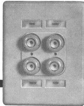
Gruppen-Sicherungselemente Type UG 3 Grössen, 2-, 4- und 6x25 A, 500 V
