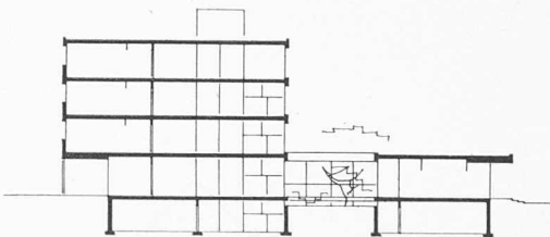
Schnitt Südwest—Nordost 1:600
