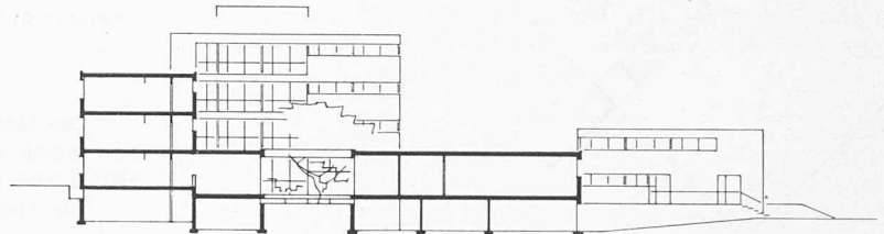
Schnitt Südost—Nordwest 1:600
