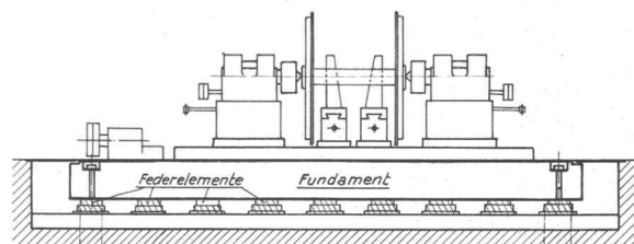
Gegen Hammerstöße passiv-entstörte Präzisionsdrehbank
