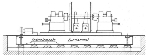
Gegen Hammerstöße passiv-entstörte Präzisionsdrehbank
