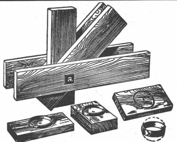
RINGDÜBEL + PATENT, Knotenpunktverbindung für hölzerne Tragwerke
