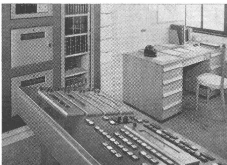
Automatenraum und Kommandopult der Betonfabrik
