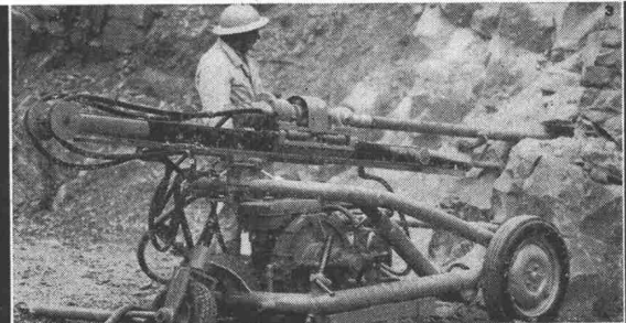
Grosslochbohrwagen mit hydraulischem Antrieb für Lochhämmer
