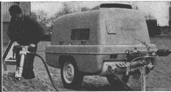
neuer, lärmärmer, vollkommen luftgekühlter 4 m 3 -Kompressor
