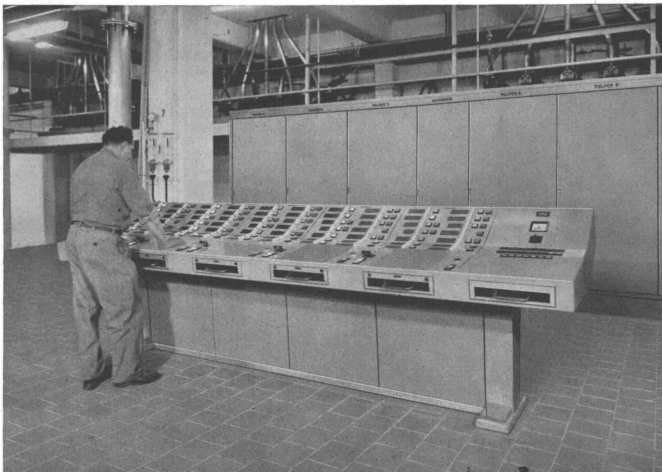
Steuerpult einer automatischen Anlage für die Papierfabrikation
