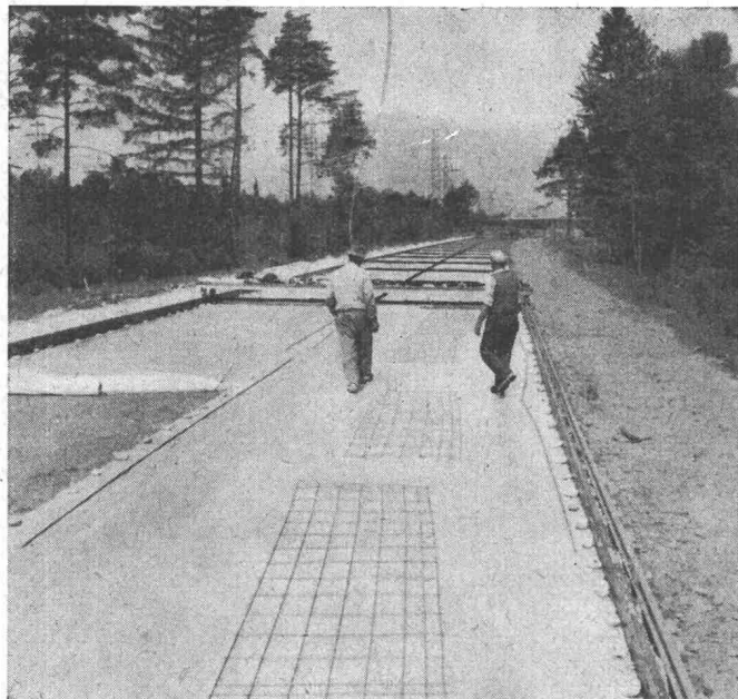
Polyäthylen «Howagaine» im Strassenbau
