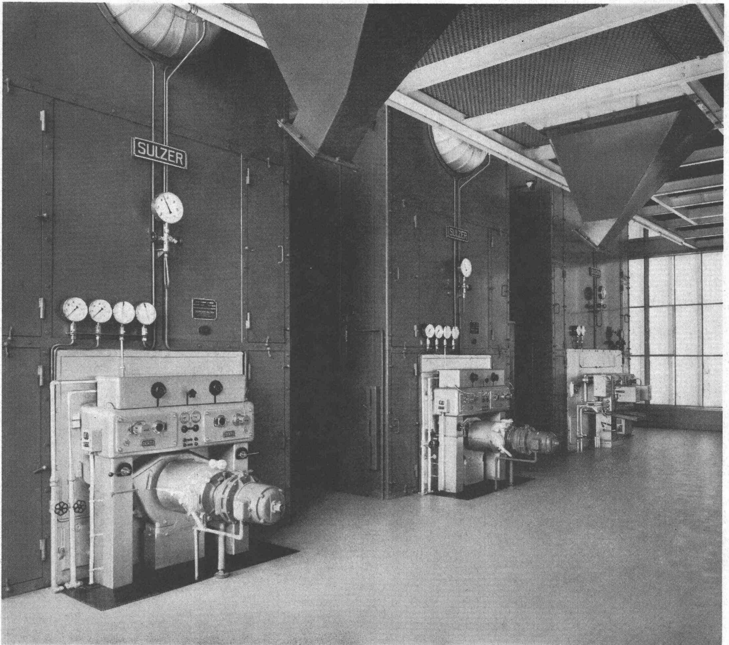
Strahlungskesselanlage der Firma F. J. Burrus & Cie., Boncourt, mit zwei Einheiten für je 1,25 Millionen kcal/h und 13 atü Betriebsdruck (vorn), mit Kohlen- und Ölfeuerung. Hinterer Kessel für 2,5 Millionen kcal/h, 15 atü und Ölfeuerung
