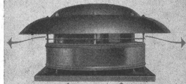
Horizontal ausblasender Entlüfter für Dachaufbau
