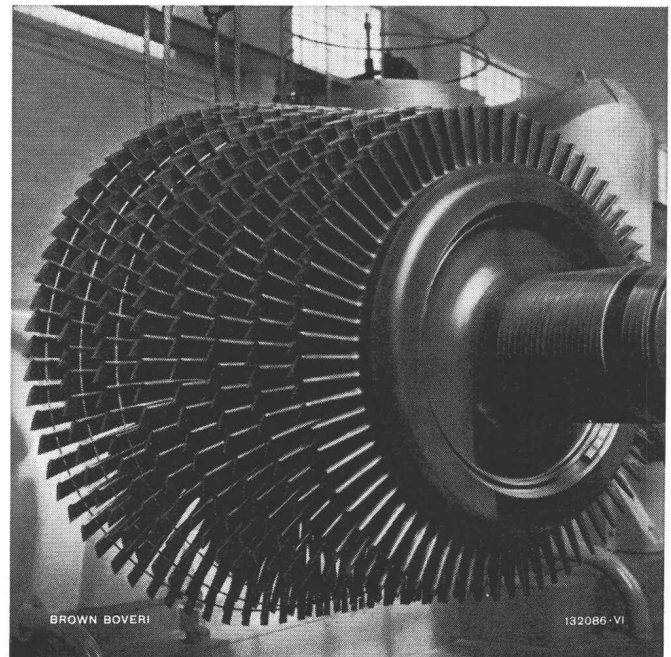
Turbinenrotor einer 5000-kW-Gasturbine
