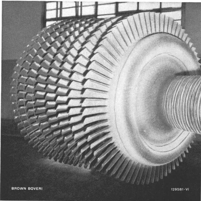
Turbinenrotor einer 5000-kW-Gasturbine
