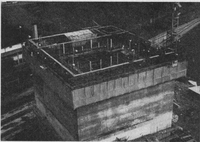
Rohwarensilo der V. L. G., Herzogenbuchsee, mit Maschinenhaus. Grundriss 20,59 × 22,84 m mit 64 Zellen und Lift, Zwischen Maschinenhaus und Zellentrakt wurde eine ausgebildete Trennfuge mitgezogen. Wandstärke: 12—20 cm. Ziehhöhen: Zellen 22 m, Aufbau über Zellen 8,07 m, Maschinenhaus 36,00 m. Betonsichtfläche: 19 000 m 2 . Erstellung vom 15. Juli bis 15. Dezember 1966
