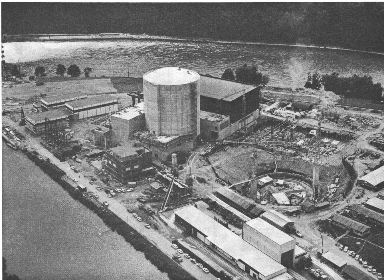
Atomkraftwerke Beznau
