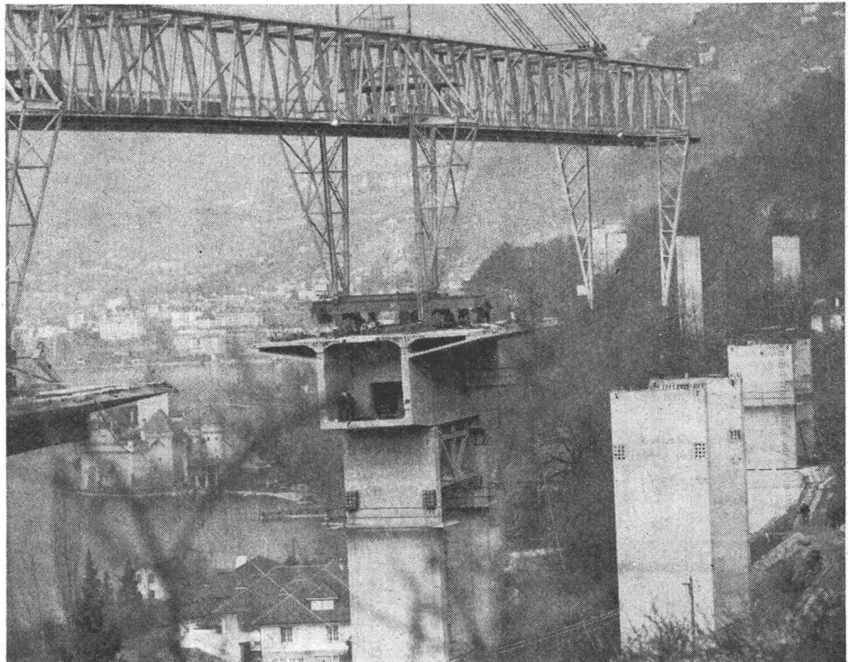
Viadukt Chillon
