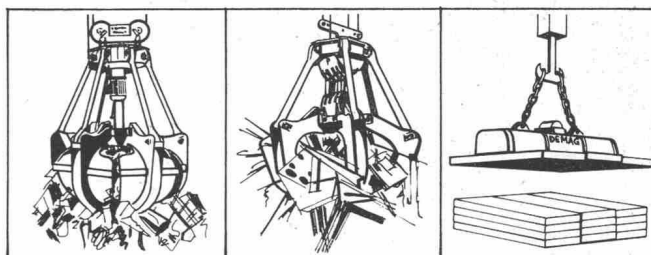
Polyp-Greifer für Kehricht
