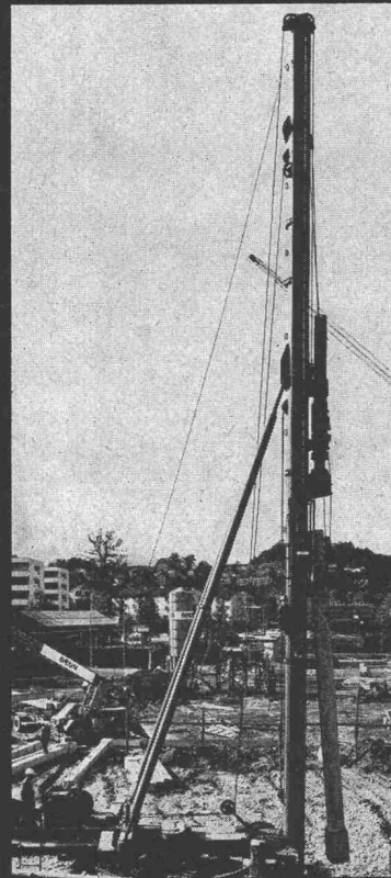
Pfählung Aalto-Hochhaus Luzern
