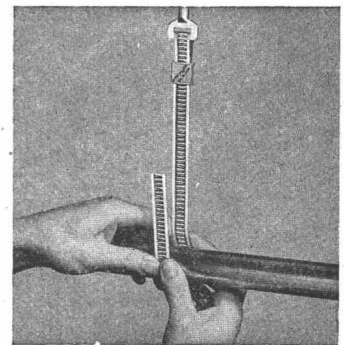
Bild 2. Langer Bandteil sauber das Rohr biegen, so dass dasselbe ganz umschlossen ist.
