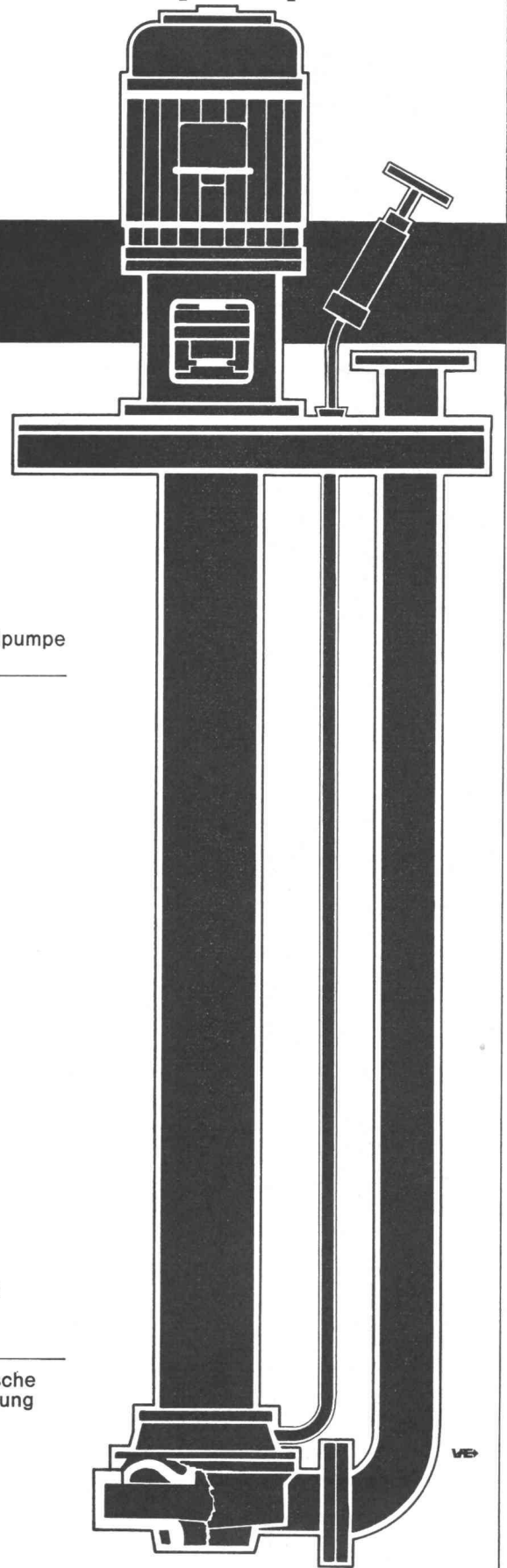
2 HÄNY-Normschacht
