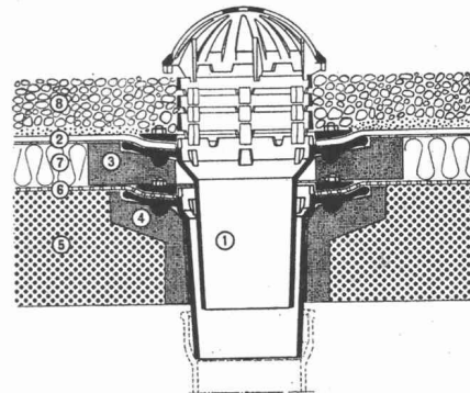
Zweiteiliger Standard-Dachablauf im Kiesschüttdach
