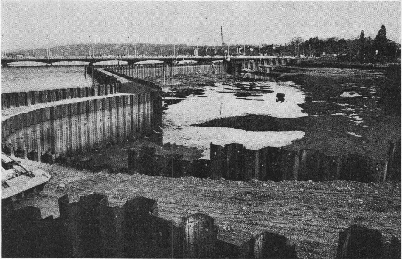
Fangdamm für die Baugrube Parking du Pont du Mont-Blanc, Genf
