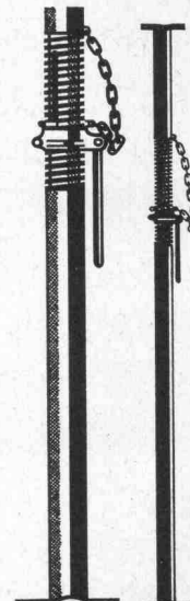
Die Deckenstütze
