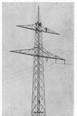
Aufgestockter 70-Meter-Mast
