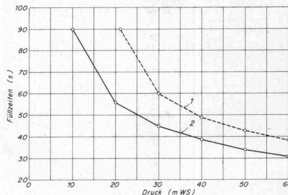
Bild 2. Geräuschentwicklung des Schwimmerventils (gemessen wurde nach DIN 52218 das durch die Leitung in den Nebenraum übertragene Geräusch). Kurve 1 Modell 1968, Kurve 2 Modell 1970
