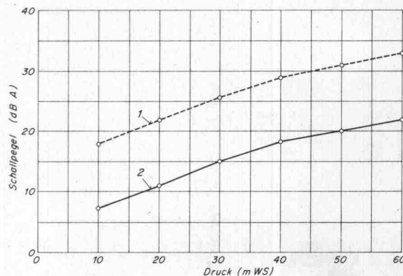
Bild 1. Zeit bis zur vollständigen Füllung des Spülkastens mit 9 l Wasser, Kurve 1 Modell 1968, Kurve 2 Modell 1970
