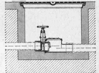
Rückstaudoppelverschluss TRIPLEX für durch- gehende Leitungen
