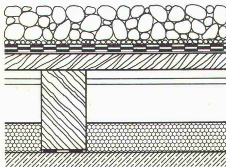
Kalddach Beispiel: Isolierung auf Stahlbetondecke
