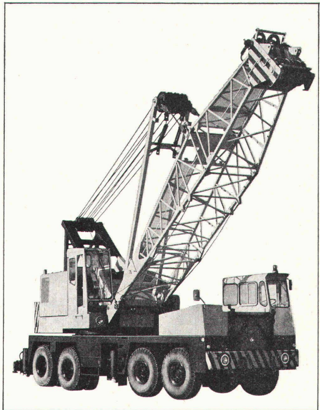
Diselelektrischer COLES-Autokran Modell Gargantua
