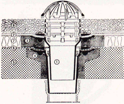
Kiesschüttdach, 2teilig
