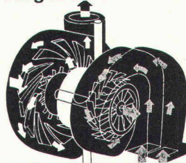
Abgasturbolader
