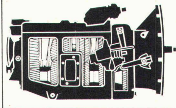
Getriebe SR 61
