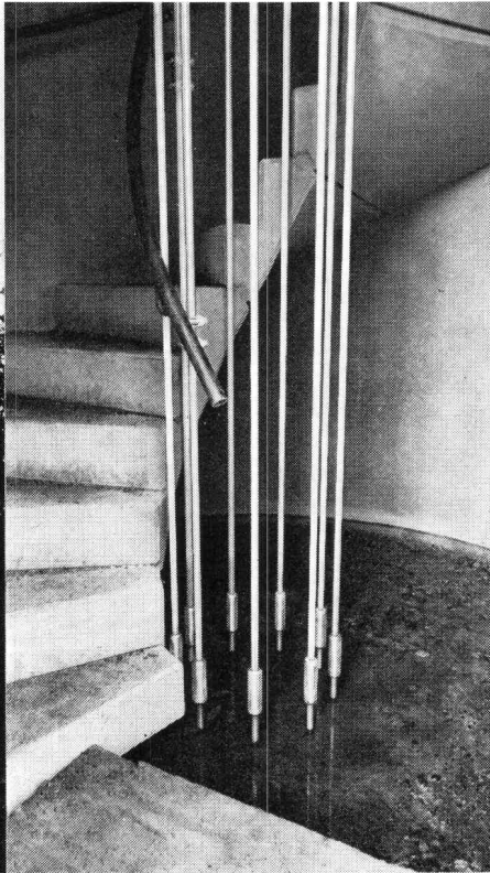
Turmvorspannung mittels gekuppelten STAIFIX-Stäben
