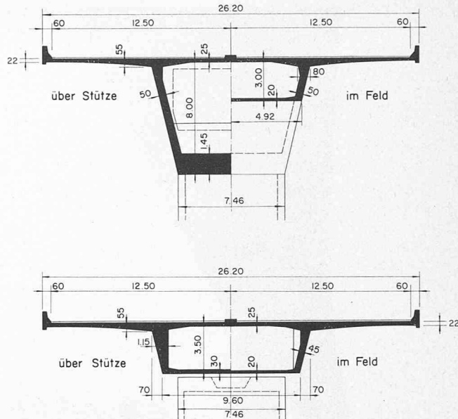
Bild 3. Brückenquerschnitte: oben Freivorbau; unten Randfelder
