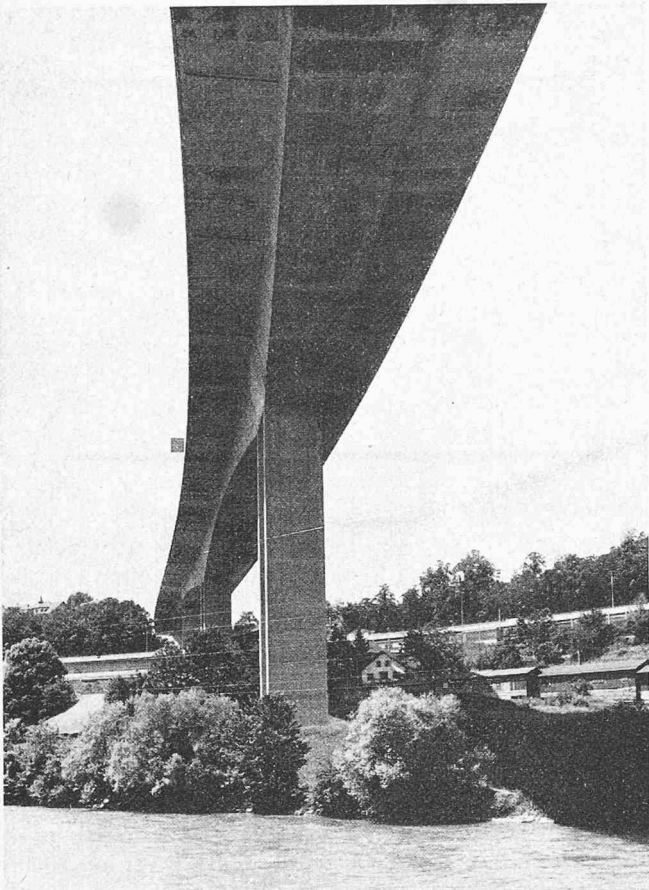
Bild 4. Brückenuntersicht
