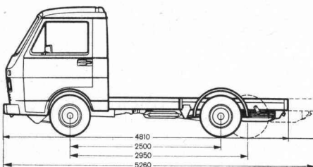
Chassiswagen.
