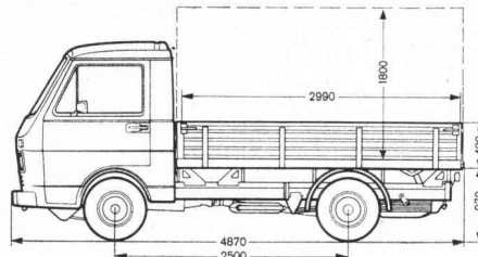
Pritschenwagen.
