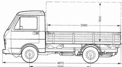
Pritschenwagen.
