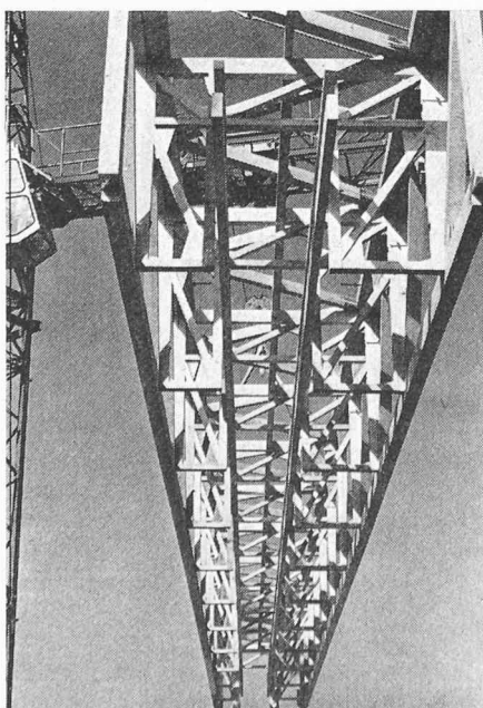
Bild 5. Vorgefertigte Bindereinheit mit eingehängtem Querrahmen für den Trennwindvorhang-Kanal und oben liegendem Wind- und Knickverband
