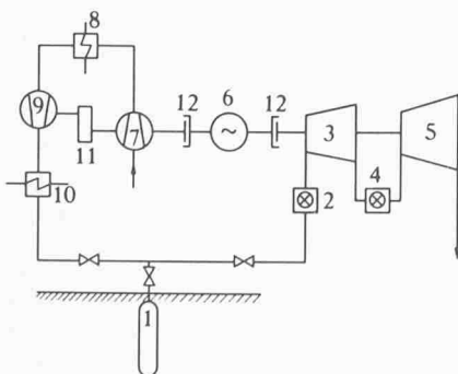
Bild 1 Schema eines Luftspeicher-Kraftwerkes
