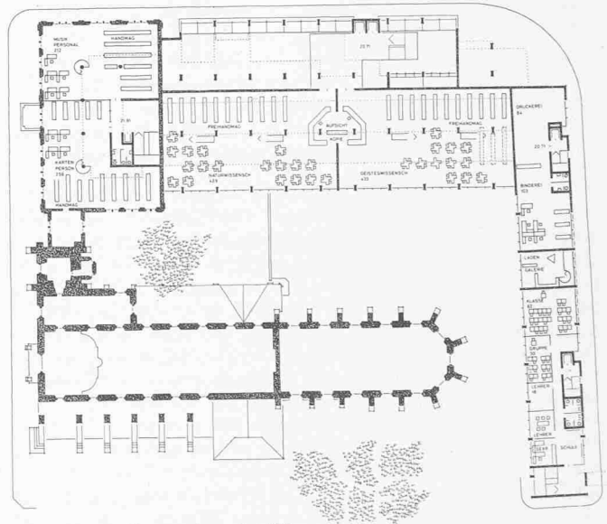
Grundriss 1. Obergeschoss 1:1100
