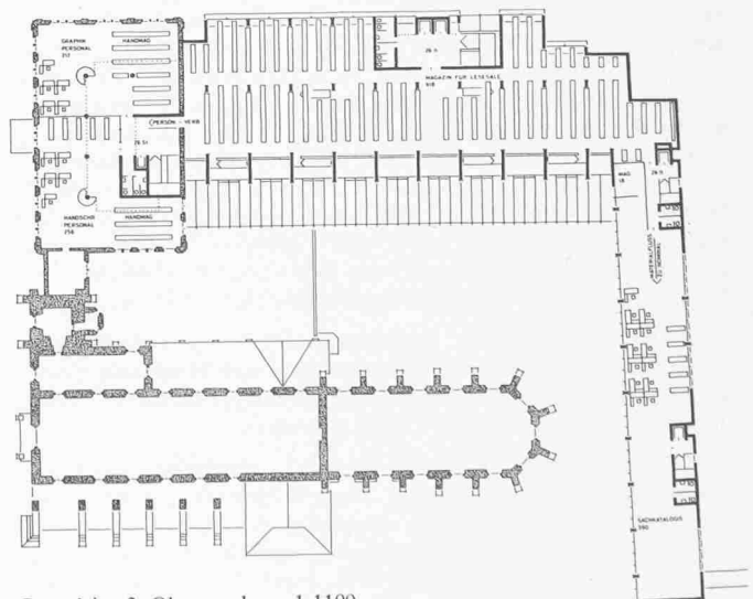
Grundriss 3. Obergeschoss 1:1100
