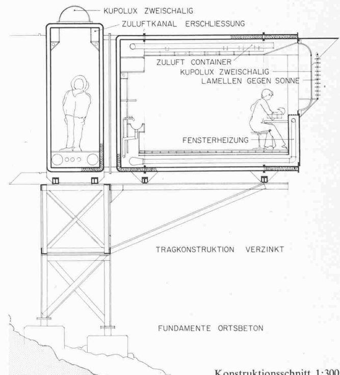
Konstruktionsschnitt 1:300
