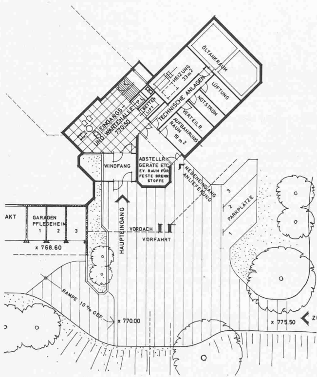
Grundriss Eingangsgeschoss 1:500
