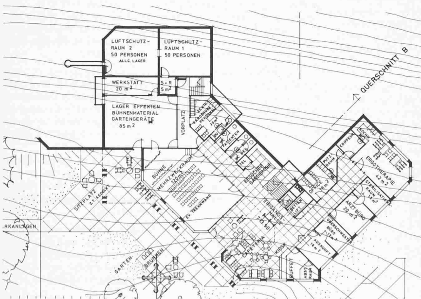
Grundriss Erdgeschoss 1:500
