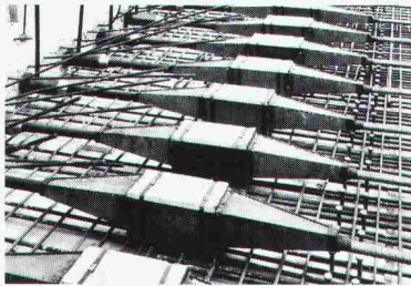
Vorfabrizierter Träger mit beweglicher Verankerung Typ A 2350
