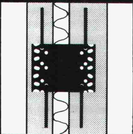
Manschettens-Verbundanker
