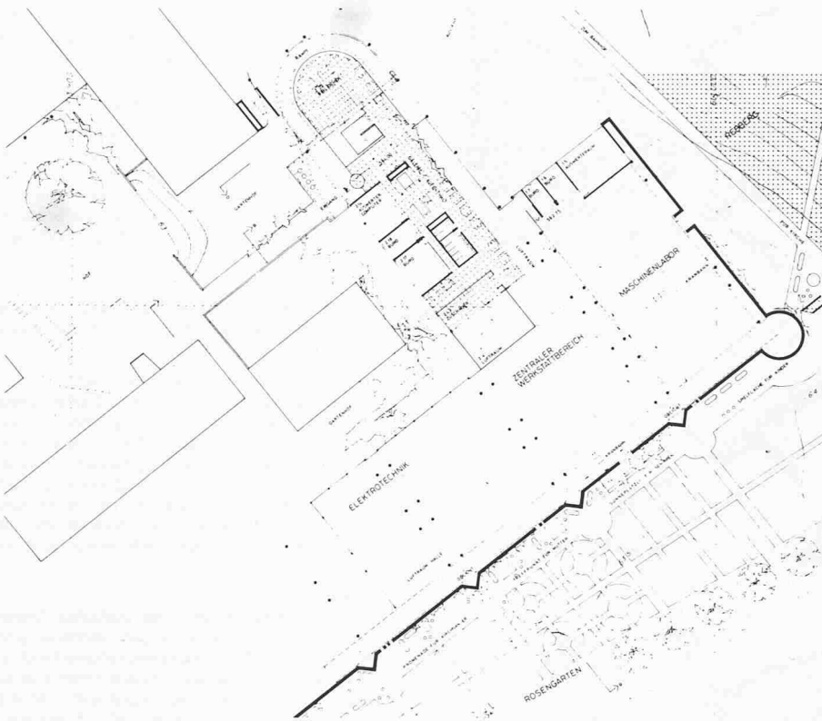
Grundriss Erdgeschoss 1 : 500
