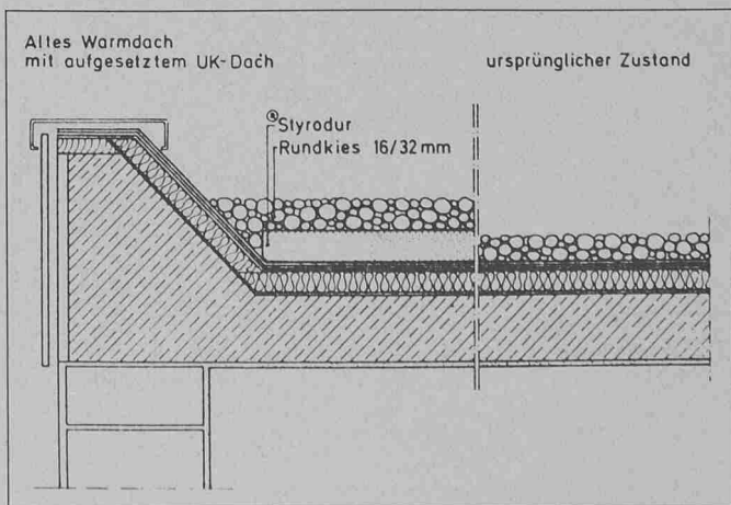
Kombiniertes Umkehrdach
