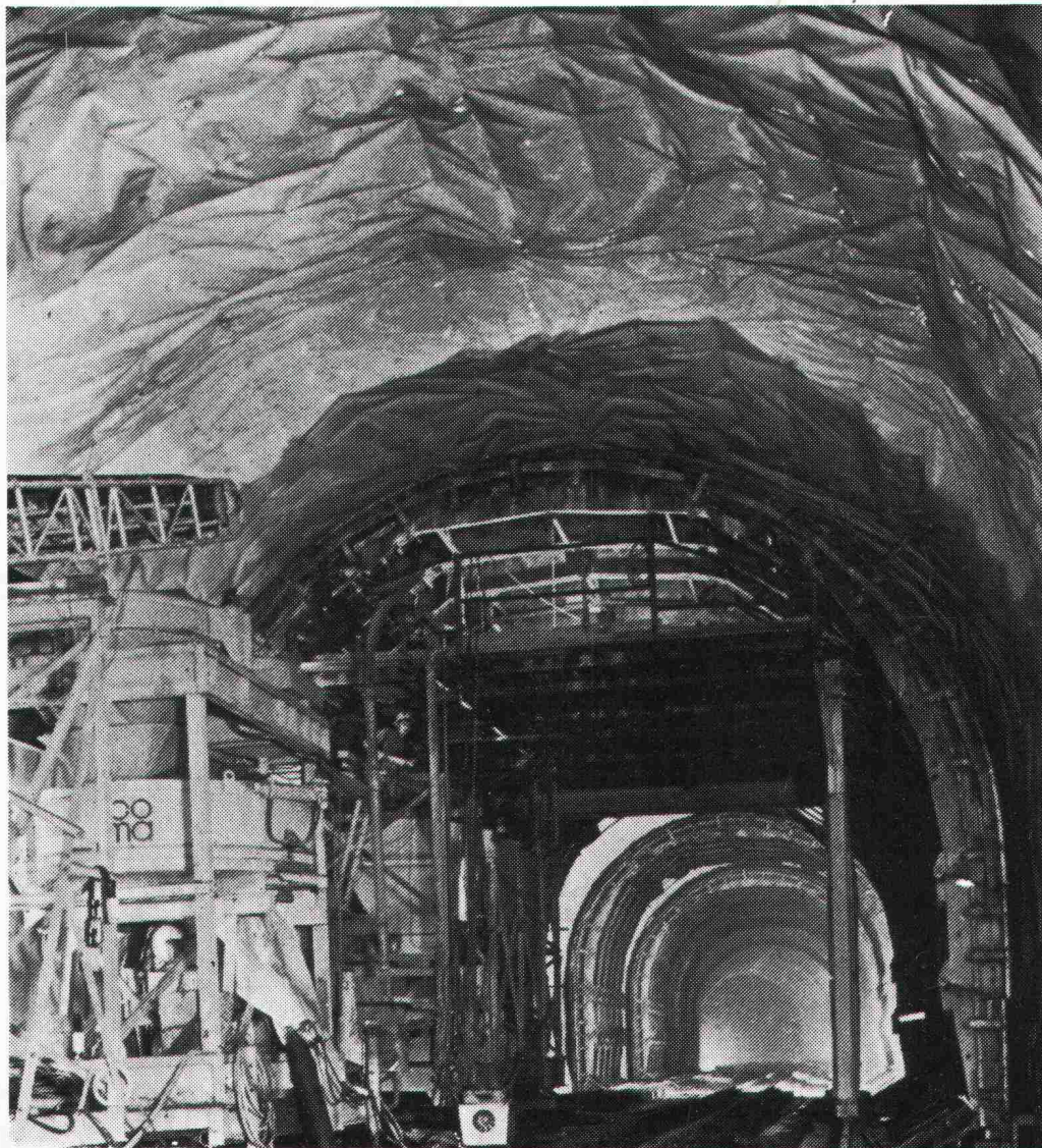
Gotthard-Strassentunnel
